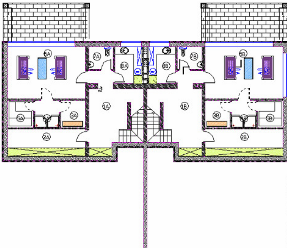
0. AUKŠTO PATALPŲ EKSPLIKACIJA
